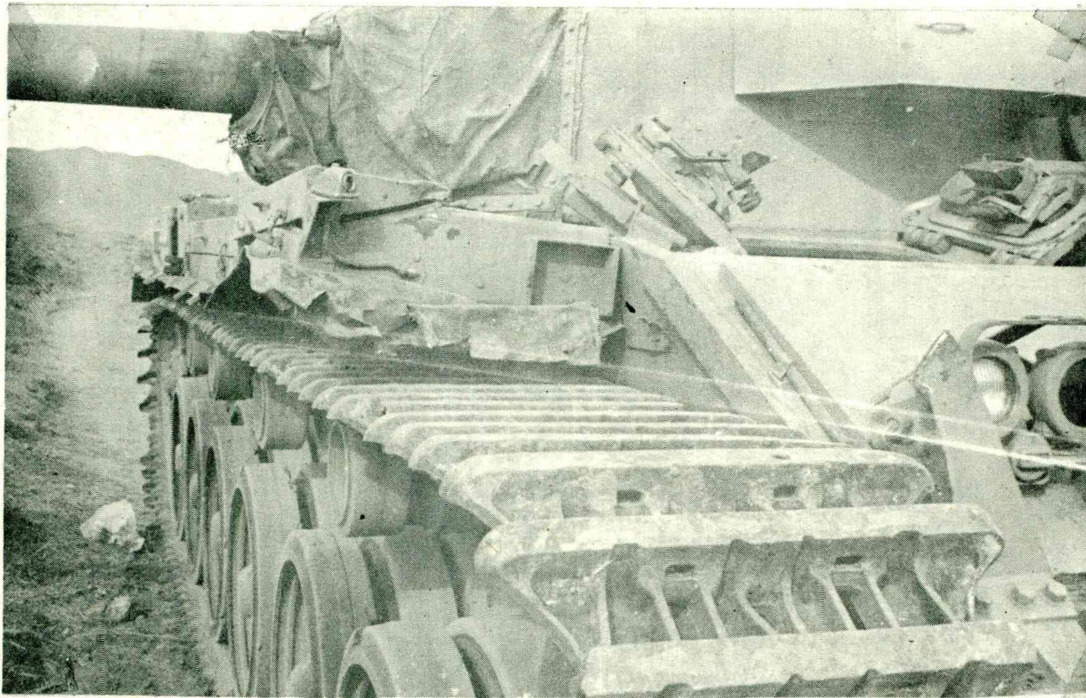
חוליות הזחל שהיו על הטנק בזמן הפגיעה.
