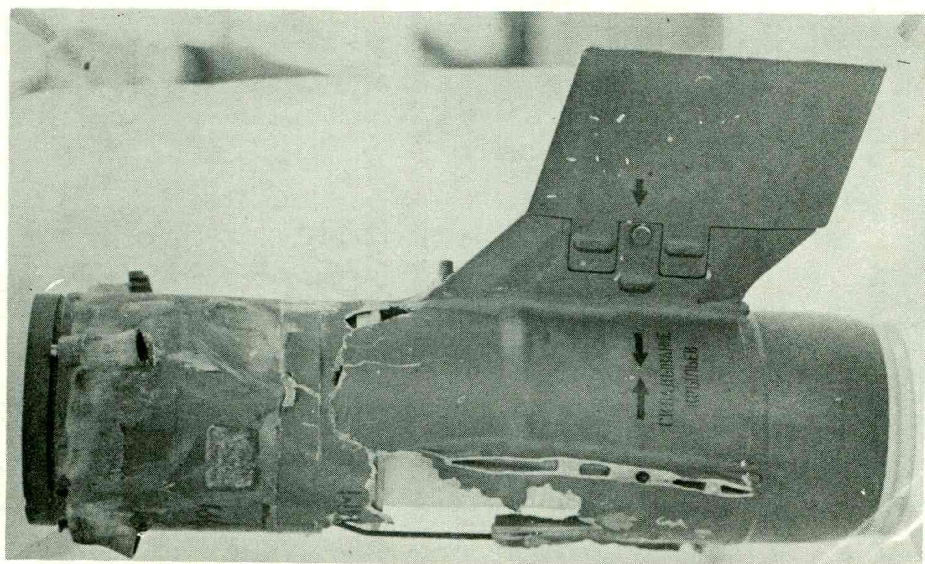
גוף הטיל וכנף יצוב פרושה.
