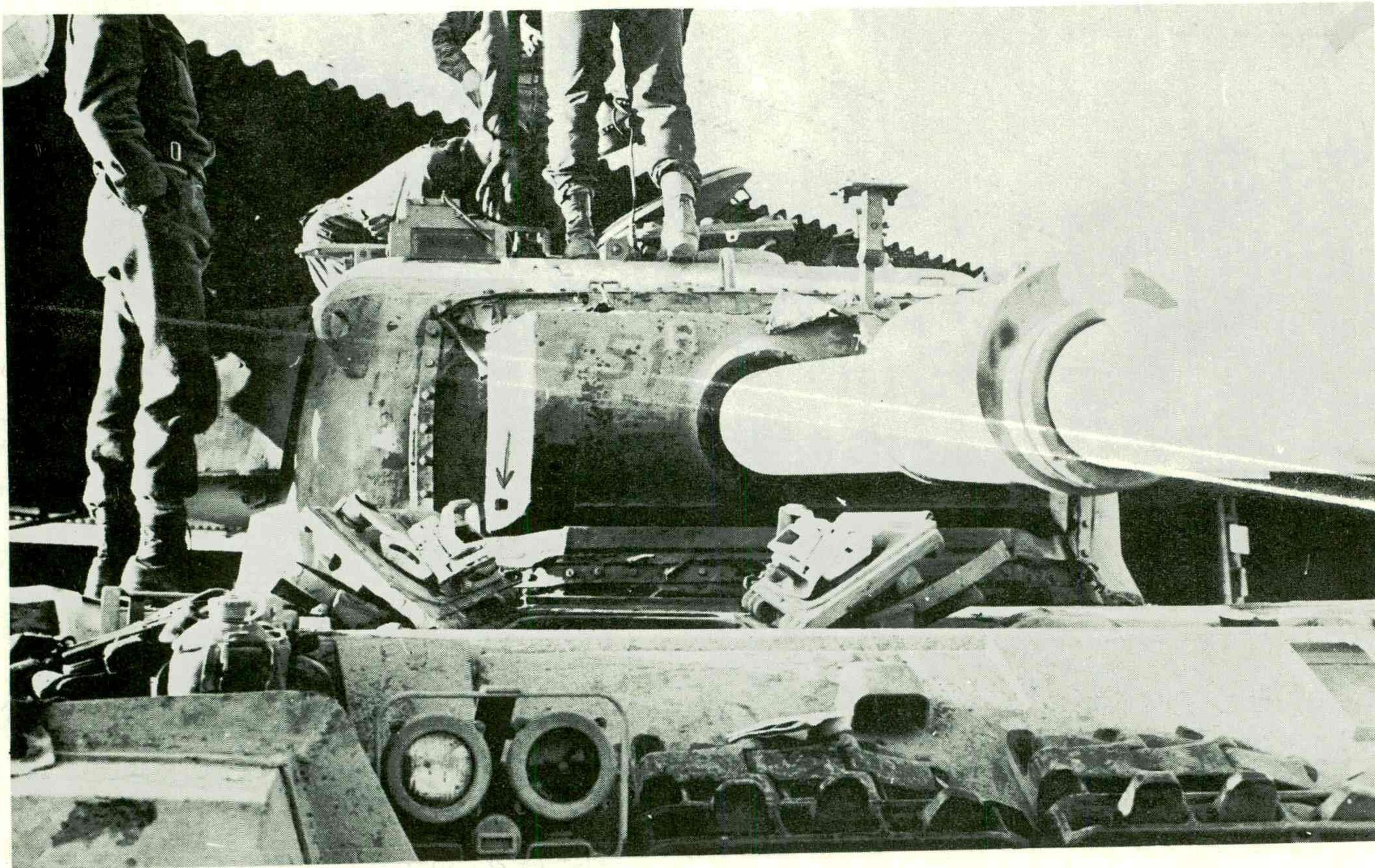
פגיעה ע"י טיל סאגר באזור מקבע התוחח. יש חדירה.
