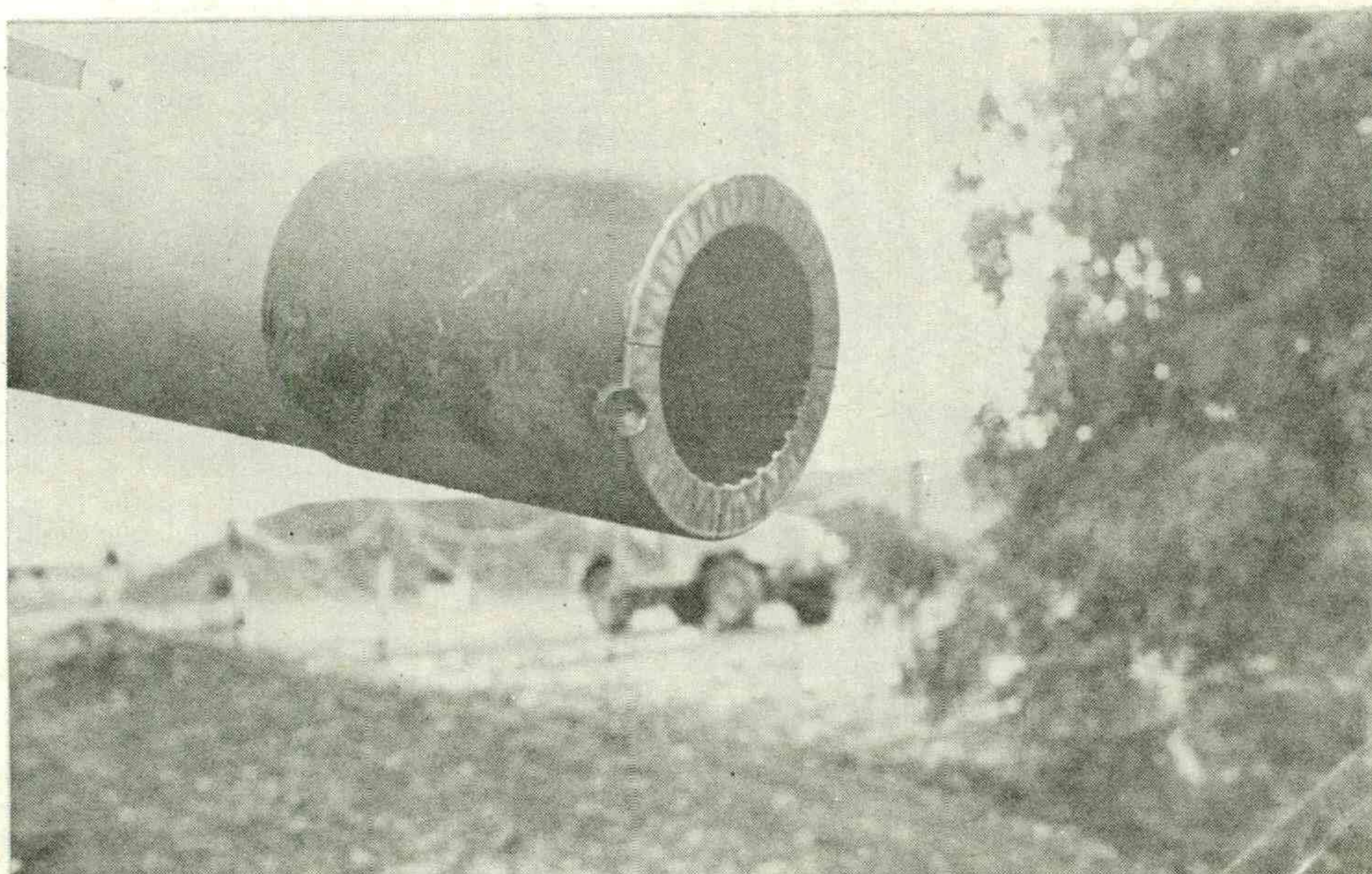
קדה הקנה נפגע מרסיס בזמן הפגיעה בטנק.
